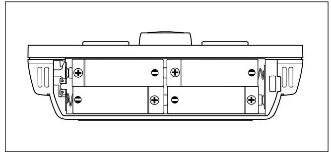
Мал. 6.6 Розташування та полярність елементів живлення
